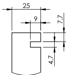
DETTAGLIO G SCALA 1 : 2
