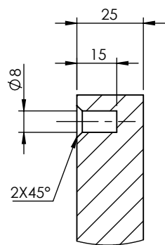
DETTAGLIO G SCALA 1 : 2
