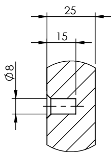
DETTAGLIO S SCALA 1 : 2
