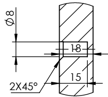
DETTAGLIO G SCALA 1 : 2
