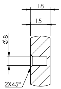
DETTAGLIO G SCALA 1 : 2
