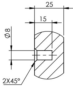
DETTAGLIO G SCALA 1 : 2
