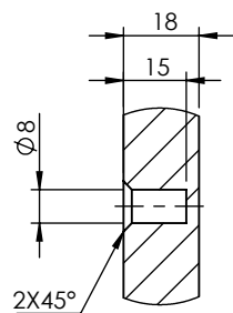
DETTAGLIO G SCALA 1 : 2
