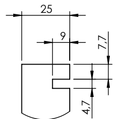
DETTAGLIO G SCALA 1 : 2
