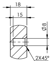
DETTAGLIO H SCALA 1 : 2
