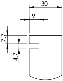
DETTAGLIO H SCALA 1 : 2
