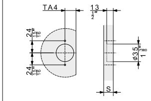
DETAIL E 2:1
