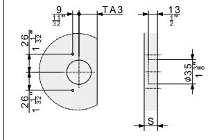
DETAIL F 2:1
