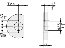
DETAIL E 2:1
