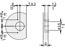
DETAIL F 2:1
