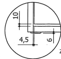
Nr. 6 piedini H.6mm regolabili Nr. 6 adjustable feet
