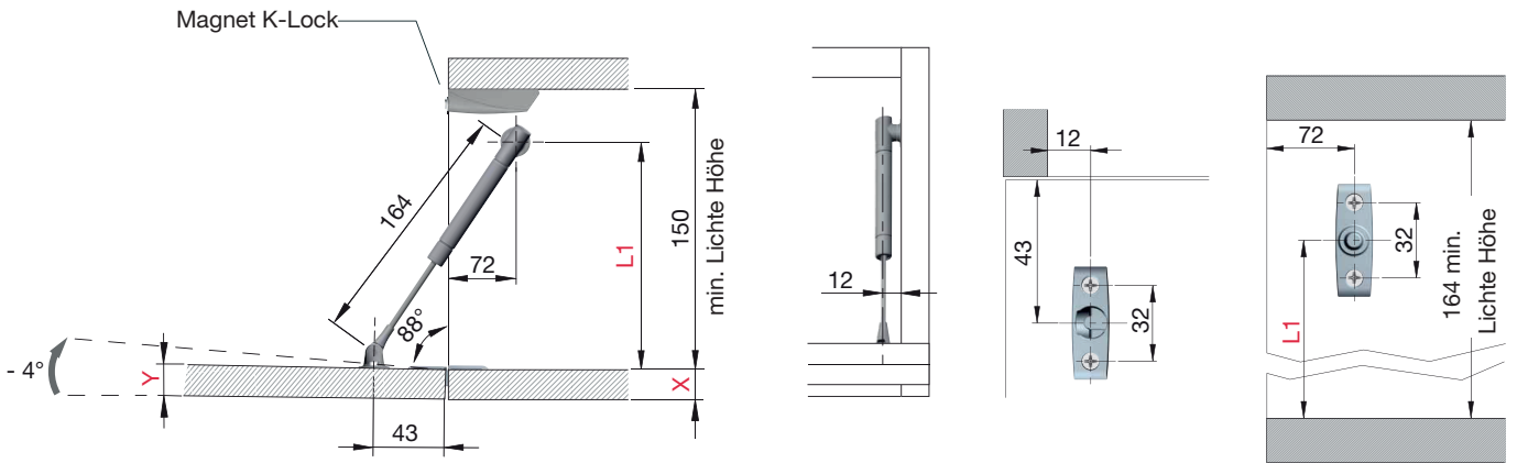
Bohrbild mit Topfscharniere ohne Push to Open
